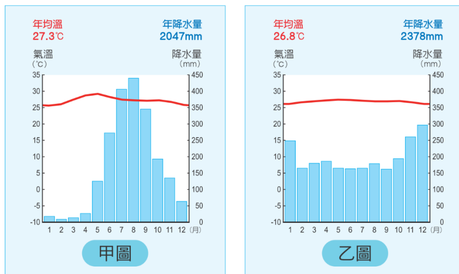
▲東南亞某兩地的氣候圖
